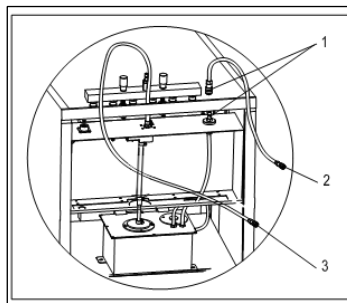
Рис. 5.16. Схема подключения
