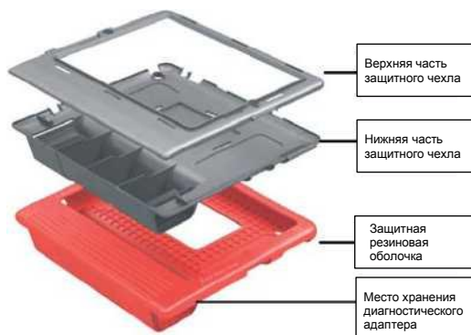
Рис. 1-3 Защитный чехол
